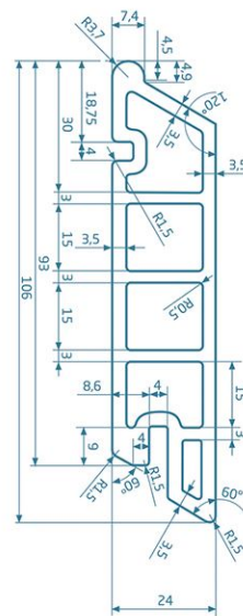
PROFIL ELEWACYJNY 106 X 24 MM
