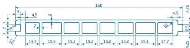
PROFIL OGRODZENIOWY 1720 X 160 X 15 MM
