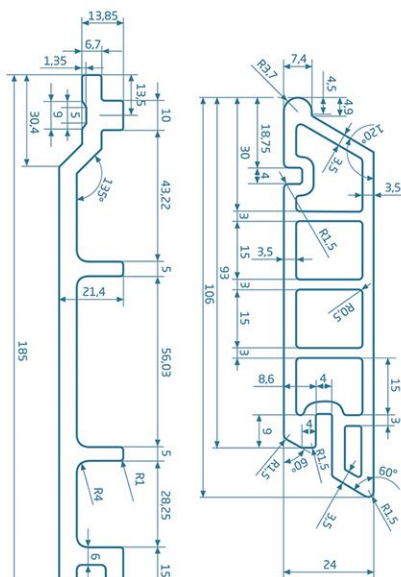
PROFIL ELEWACYJNY 106 X 24 MM
