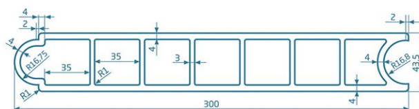
PROFIL OGRODZENIOWY 1950 X 300 X 43,5 MM
