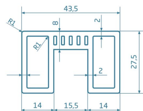
LISTWA OGRODZENIOWA C 1750 X 27,5 X 43,5 MM
