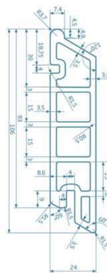
PROFIL ELEWACYJNY 106 X 24 MM
